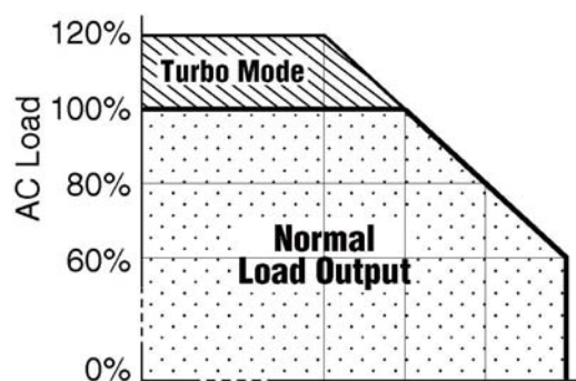
出力負荷 / 温度ディレーティングと ターボモード
