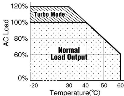
出力負荷 / 温度デレーティングとターボモード
