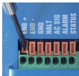
橙色の開閉用ボタンを押し込みます。
