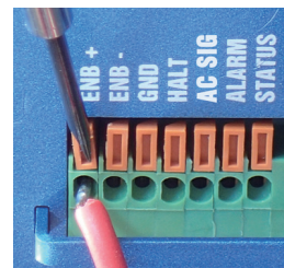
ケーブルを奥まで挿入戻すと固定されます。
